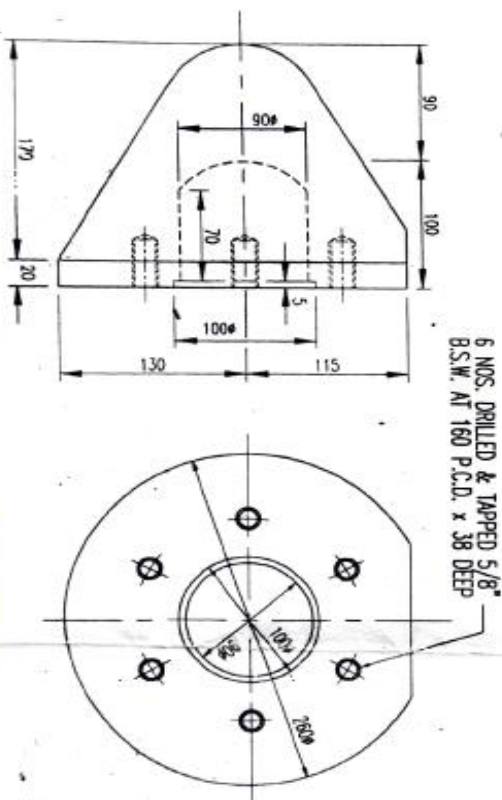
CAST IRON CONE (PART NO: 50)
